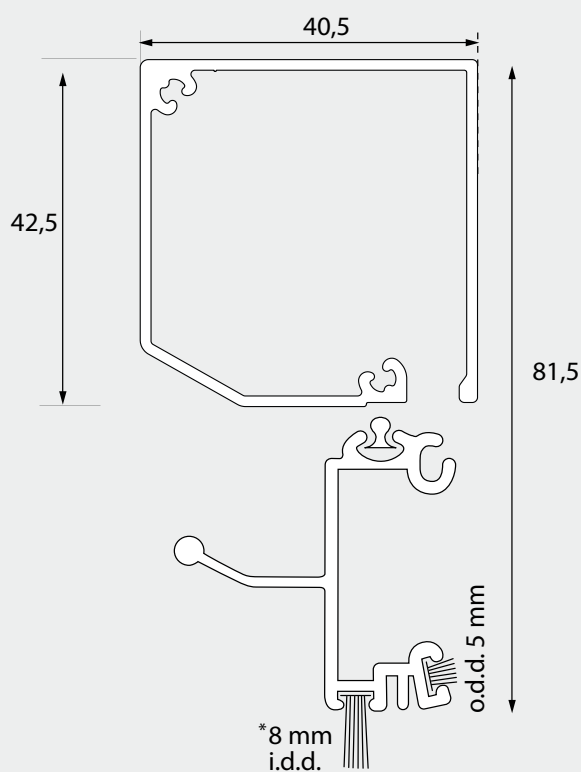
Doorsnede:
