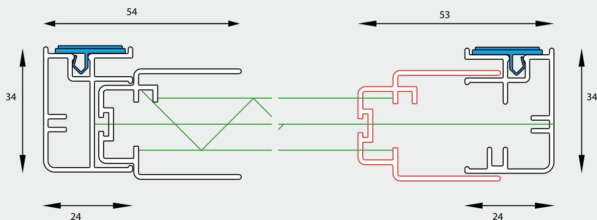
Doorsnede:
