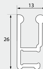
Glijrail:
