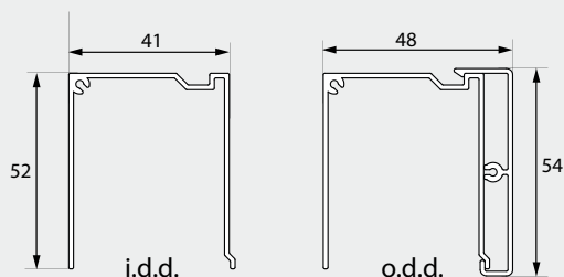
U-profiel (bovengeleider)
