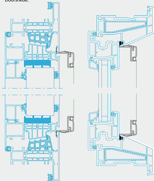
ALUMINIUM kozijn dagmaten opgeven
