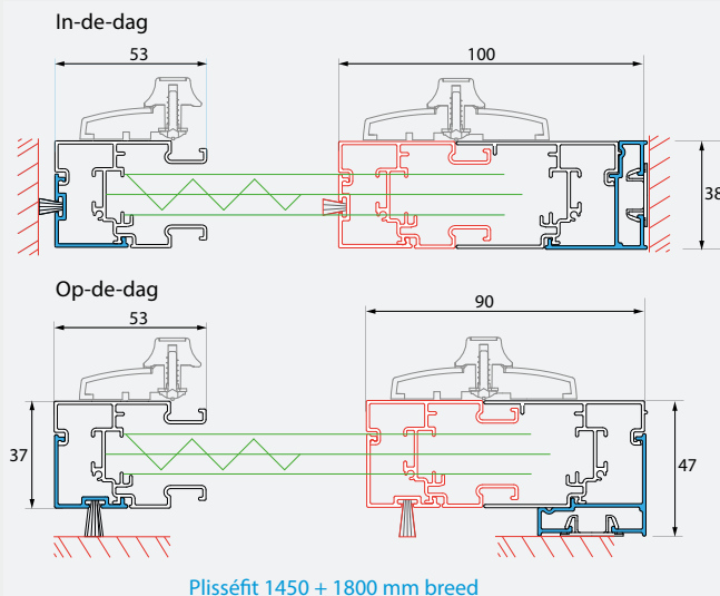
Plisséfit 1450 + 1800 mm breed
