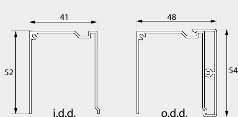
U-profiel (bovengeleider)
