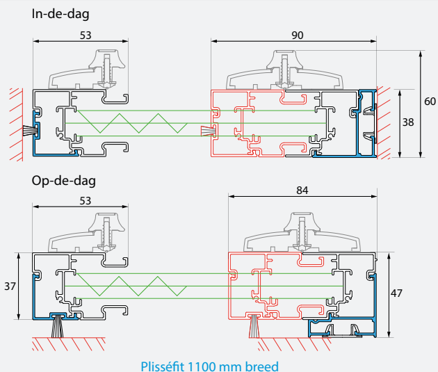
Plisséfit 1100 mm breed
