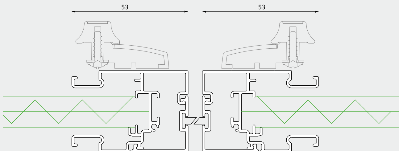
Dubbele Plisséfit met magneetsluiting
