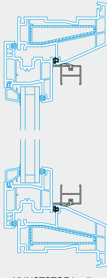
KUNSTSTOF kozijn Dagmaten opgeven
